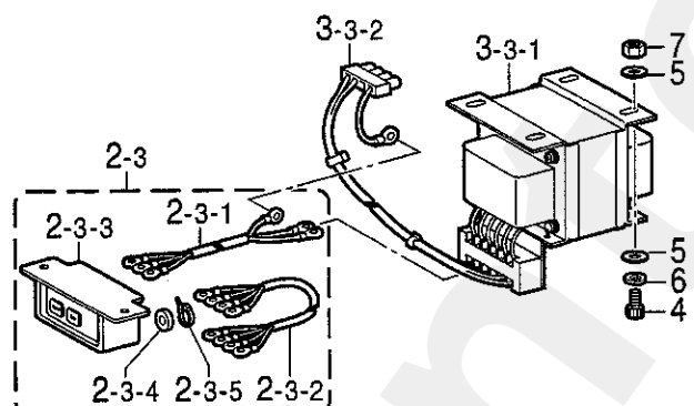
< 三相400V (ヨーロッパ) / For "3-Phase 400V AC (EUR)" >
