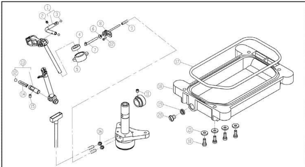
二十一、供油机构(2)/Lubrication Mechanism(2)
