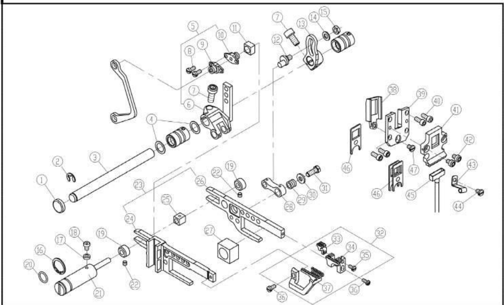
十七、送布机构/Feed Mechanism
