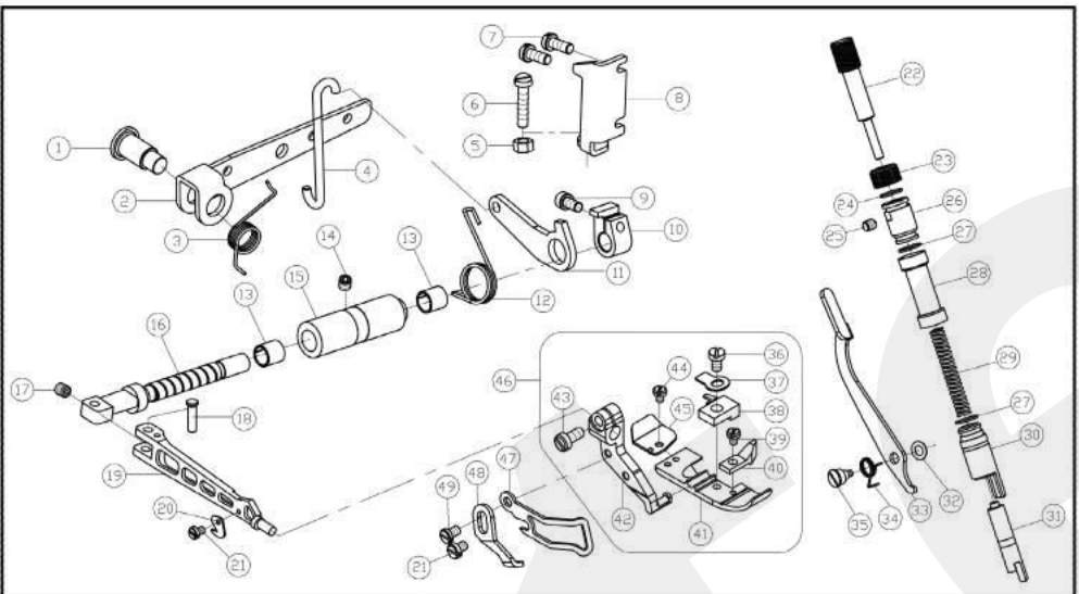
十九、抬压脚机构/Presser Foot Mechanism
