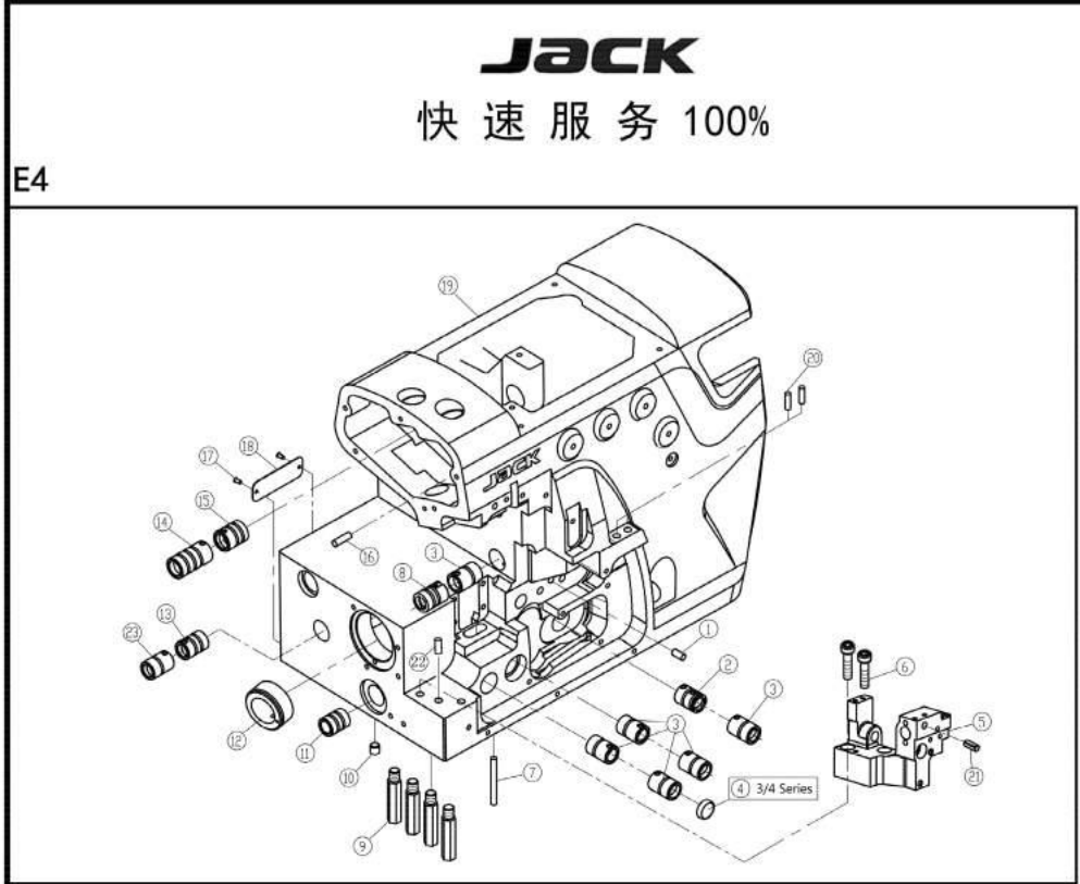
一、机壳部分/Machine Bed Frame
