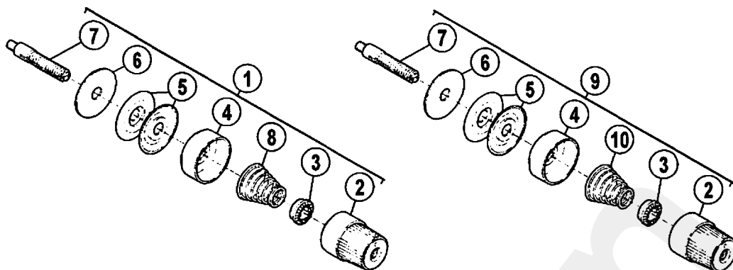
■1本針(1-needle) EX5203・5204・5205
